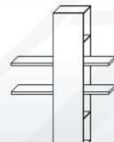
Полка навесная «Альда» КМК 0782.10 1300*1805*400
