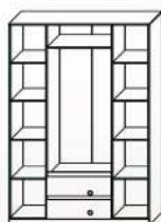
Шкаф «4Д2Я Николь» КМК 0683.13 1605*2300*580
