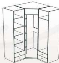
Полка «Угловая Б» КМК 0320.4 300*2195*560
