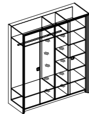
50.300 Шкаф для одежды 2204x1947x651
