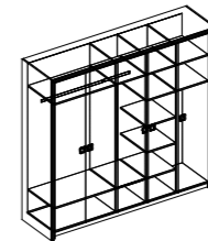
50.315 Шкаф для одежды 2204x2393x651
