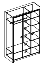
50.302 Шкаф для одежды 2204x1501x651
