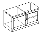
Кт 35.110 Тумба 2 дв. 506×899×428
