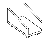
Кт 35.700 Подставка под системный блок 283×294×500
