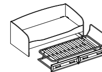
Кт 35.355 Кровать 2-х местная 804×1960×962
