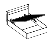
Кт 35.335 Кровать 900×1500×2109
