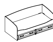
Кт 35.350 Кровать 2 ящ. 804×1960×962
