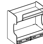
Кт 35.370 Кровать двухъярусная 2 ящ. 1866×1972×962
