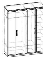
Лт 36.661 Шкаф для одежды 2360x1794x628
