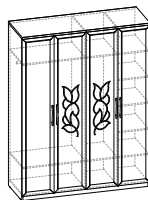
Лт 36.660 Шкаф для одежды 2360x1794x628
