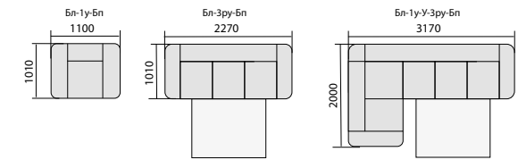
Механизм «Седяфлекс» Спальное место 1540x1950 мм
