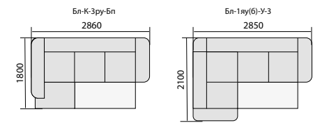
Бл-К-Зру-Бп Механизм «Дельфин» Спальное место 2300x1450 мм
