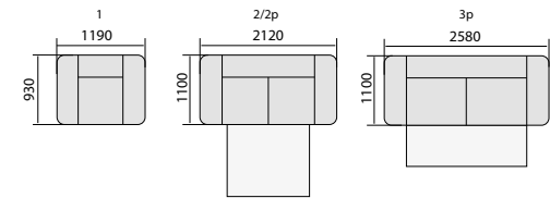
2р — механизм «Французская раскладушка» Спальное место 1770x1300 мм
