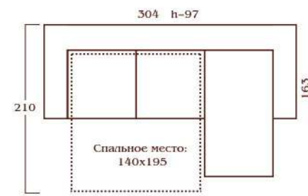
Римини Диван-кровать с шезлонгом. 1. Механизм «дайтон».
