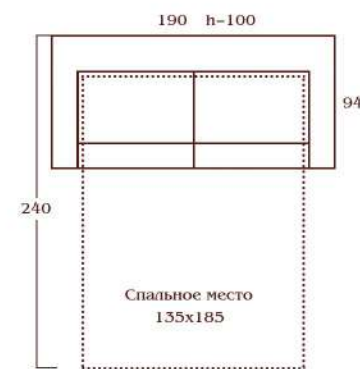
Глория-05 Диван-кровать двухместный тахі, прямой. 1. Механизм «3 сложения».
