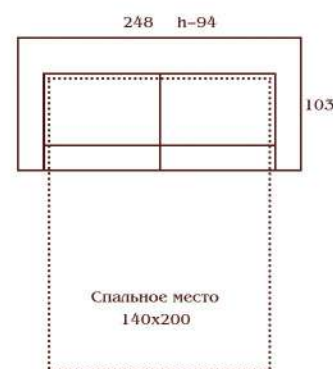
Неаполь Диван-кровать трехместный, прямой. 1. Механизм «дельфин».
