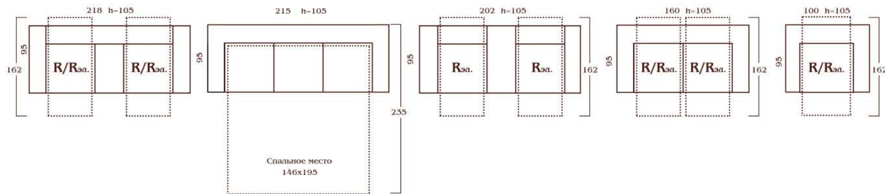
Тоскана Диван трехместный, прямой, два механизма «реклайнер»/«электрореклайнер».
