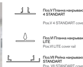
элементы облицовки lining elements
