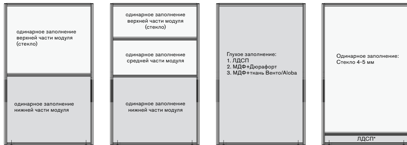
Модуль комбинированный «NAYADA-UNO»
