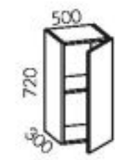
Шкаф навесной 500
