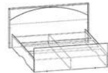
Кровать двуспальная Ш1800xВ900xД2000 Матрац 1600x1950
