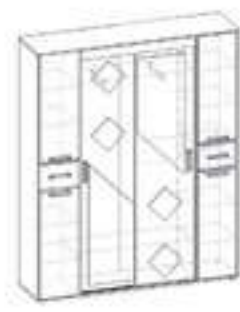
Шкаф-купе Алиса-3 Ш1797xВ2138xГ481
