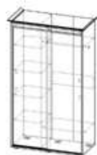
Шкаф-купе 2-х дверн. с фальцем Ш1292xВ2140xГ624
