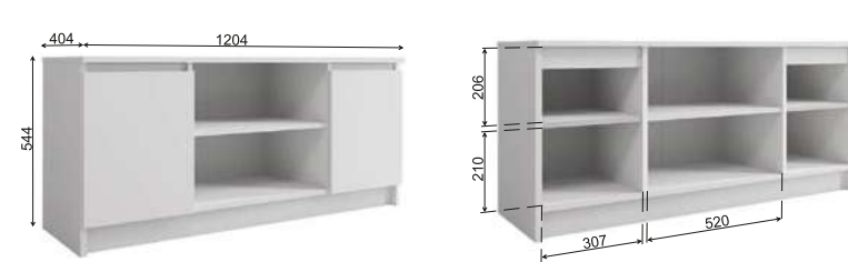
Модуль «Мори» МТВ 1200.1
