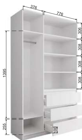
Модуль «Мори» MSHU 960.1
