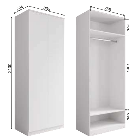
Модуль «Мори» MSH 800.1
