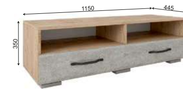
Модуль «Асти» АТБ 1150.2
