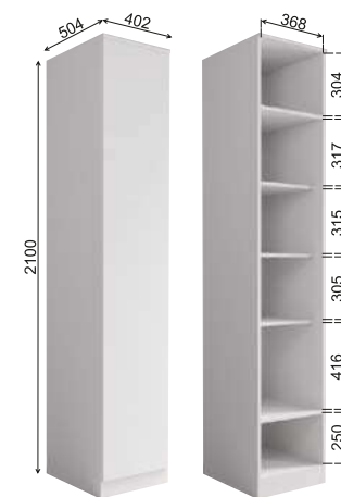
Модуль «Мори» MSH 400.1
