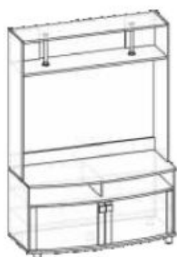
Модуль №13 1200x1688x440
