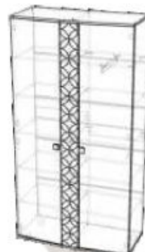
Модуль №26 1000x1966x440
