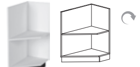
Шкаф-стол скошенный открытый к столам с гл. 525 мм. и с гл.370 ВхШхГ 820x300x525 ВхШхГ 820x300x370
