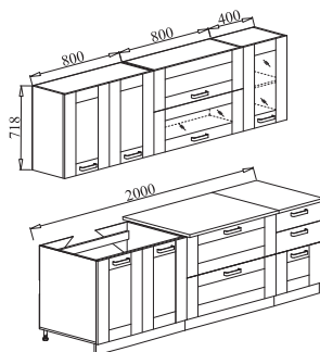
Компоновка 2,0 м.
