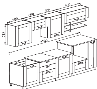
Компоновка 2,7 м
