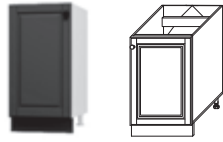
Шкаф-стол кухонный одnodверный под мойку к столам с гл. 370мм. ВхШхГ 820x500x370 ВхШхГ 820x600x370
