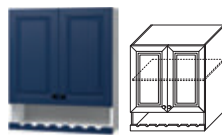
Шкаф кух. настен. 2-хдверный с полкой и нишей(декор. планка)
