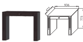
СТОЛ ТУАЛЕТНЫЙ ДхВхШ: 936x773x422 мм.
