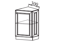
Шкаф-стол однодверный (окончание) скошенный
