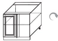
Шкаф-стол кухонный 1дверный рабочий К столам с гл. 370мм. ВхШхГ 820x800x525
