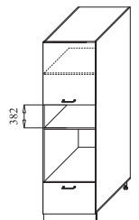
шкаф-хозяйственный под технику В6
