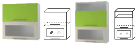
Шкаф навесной с 2-мя откидными дверями В*Ш*Г 718*600*320 В*Ш*Г 718*800*320
