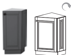
Шкаф-стол 1дверный (окончание) скошенный В*Ш*Г 820x300x370
