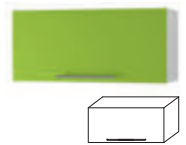
Шкаф кухонный навес- ной с откидной дверью В*Ш*Г 300x600x320 В*Ш*Г 400x600x320
