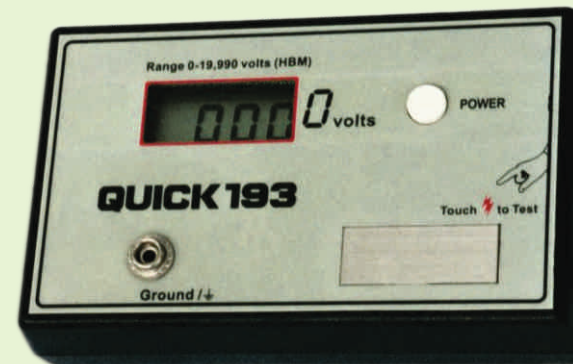
Измеритель статического напряжения QUICK 193
