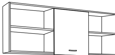
Полка (2000) (500*2045*300)
