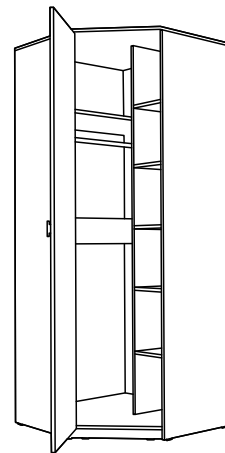
Шкаф угловой ШОУ-3м (2 150 x 850 x 500)
