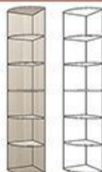
Т-52 (полки): ш. 370 / гн. 370 / выс. 2080;
