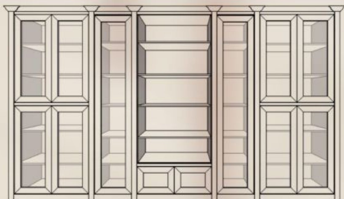
Екатерина Премиум. Библиотека на базе НКМ 1. Широкая пилястра. 2252 x 4006 x 455 (ВxШxГ)
