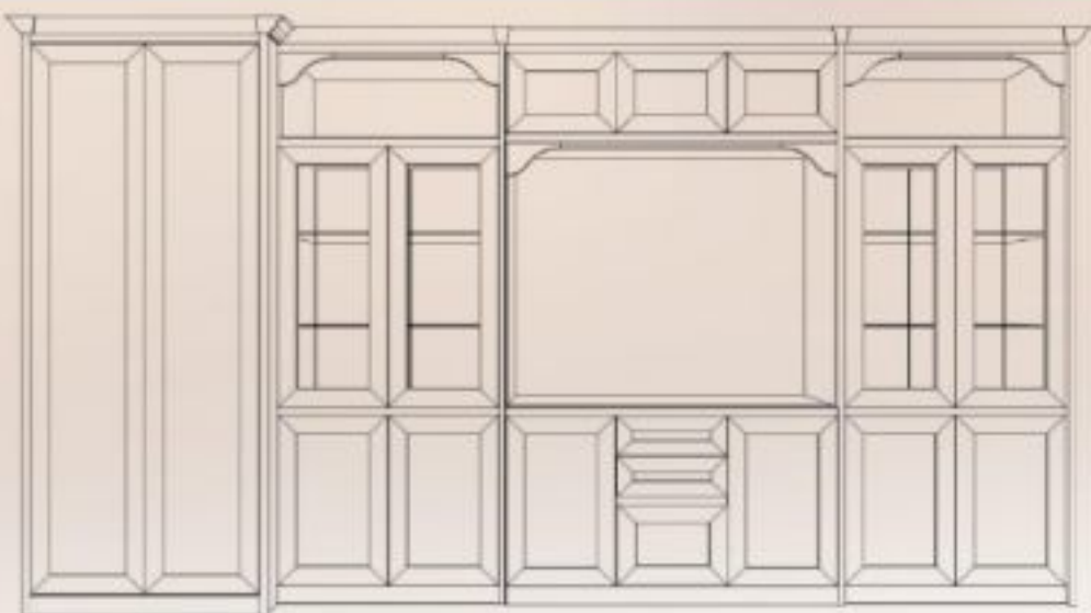
Екатерина Премиум 9. Узкая пилястра. Дуб. 2252 x 4189 x 635 (ВxШxГ)
