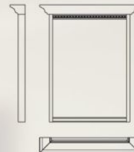
Зеркало. Красное дерево. 814 x 694 x 107 (ВxШxГ)
