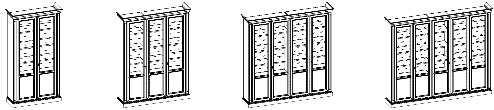
Art. 950 Библиотека 2х дверная L.113 Н.210 P. 41 V.0,36
