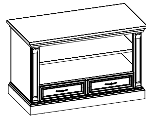
Art. 705 Тумба ТВ L.111 H.70 P.56 V.0,59
