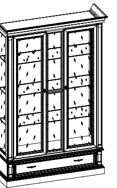
Art. 519 Витрина 2х створчатая с зеркалом и подсветкой L.134 H.210 P.45 V.1,53
